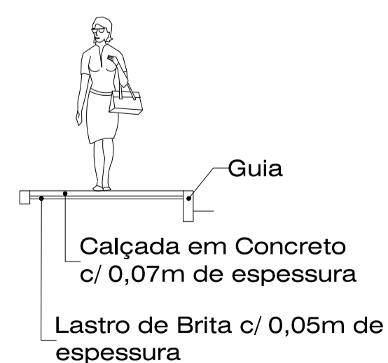
PASSEIO PUBLICO - CORTE AA ESC: 1:20
