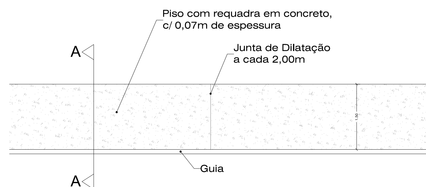
PASSEIO PUBLICO ESC: 1:20
