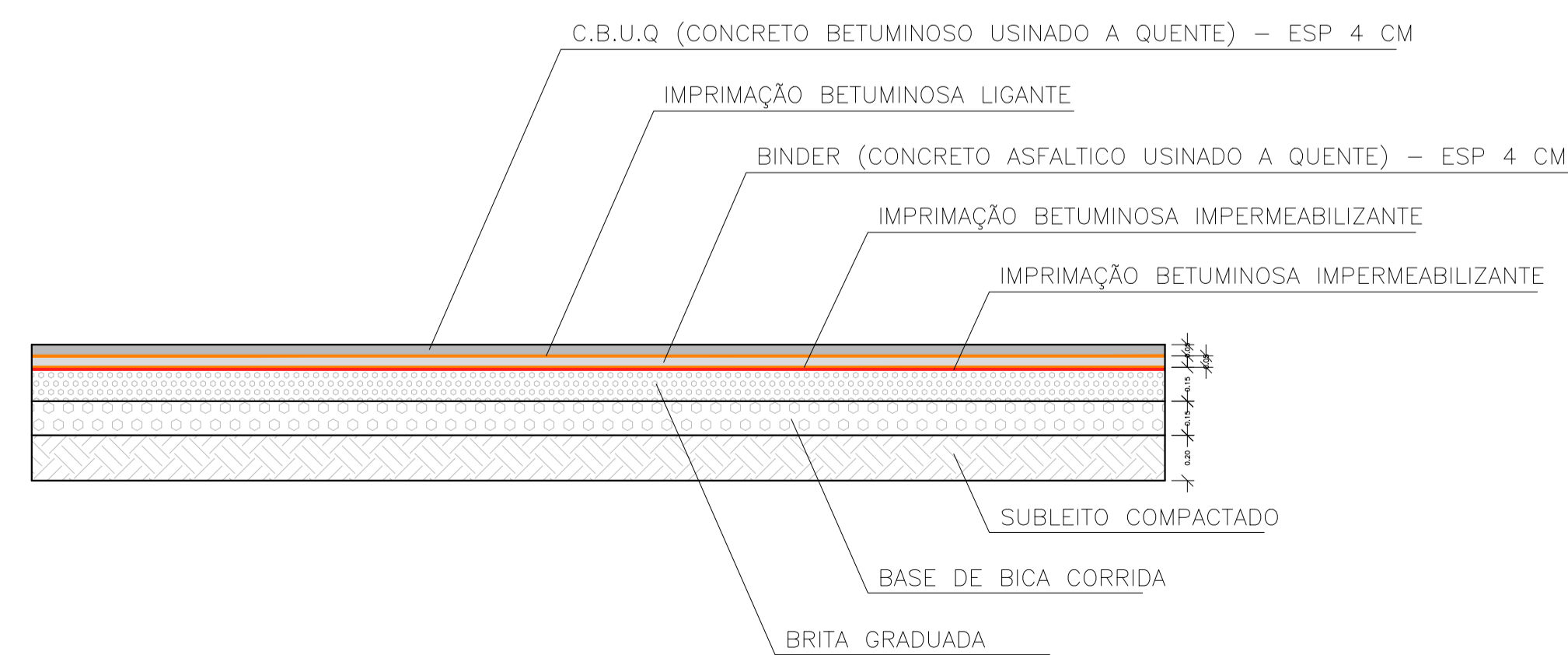
CORTE PAVIMENTAÇÃO ESC: 1:20
