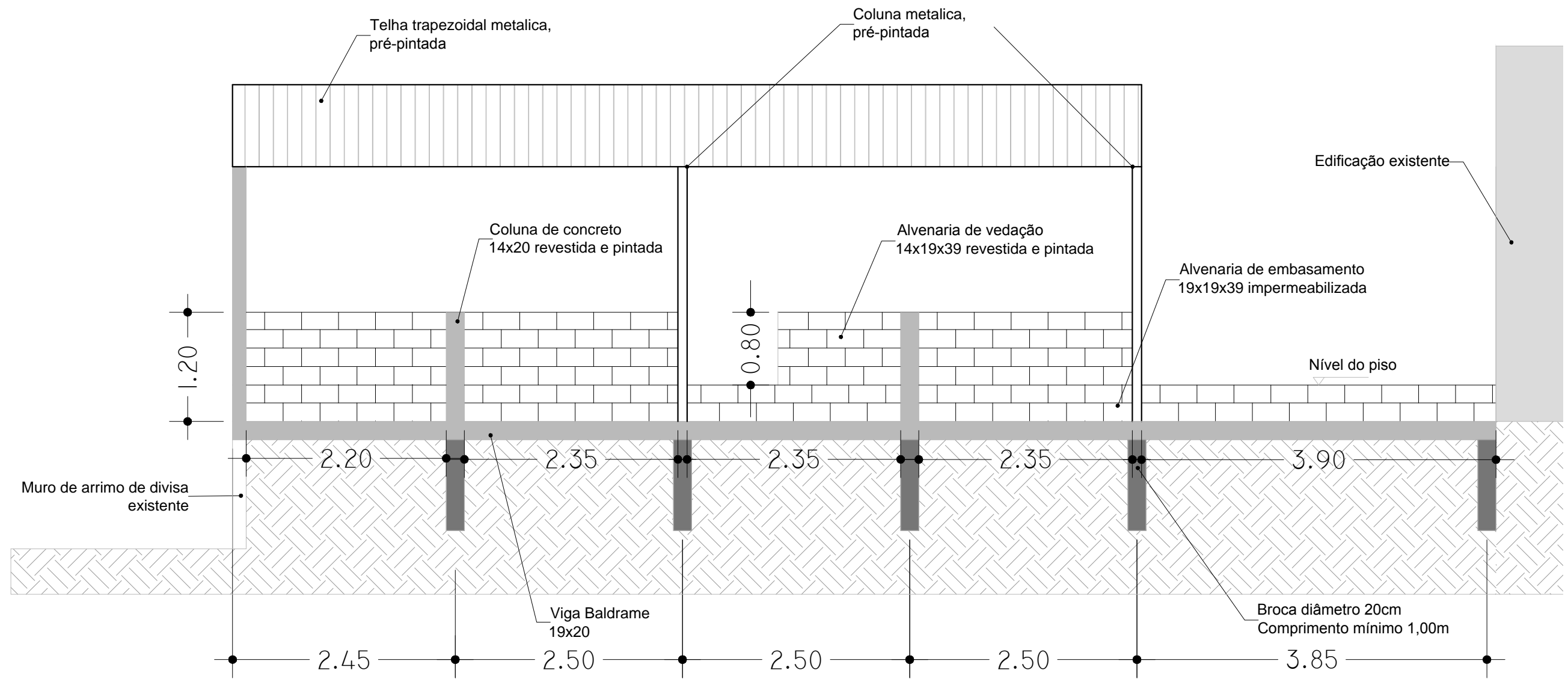
VISTA BB ESCALA 1:50
