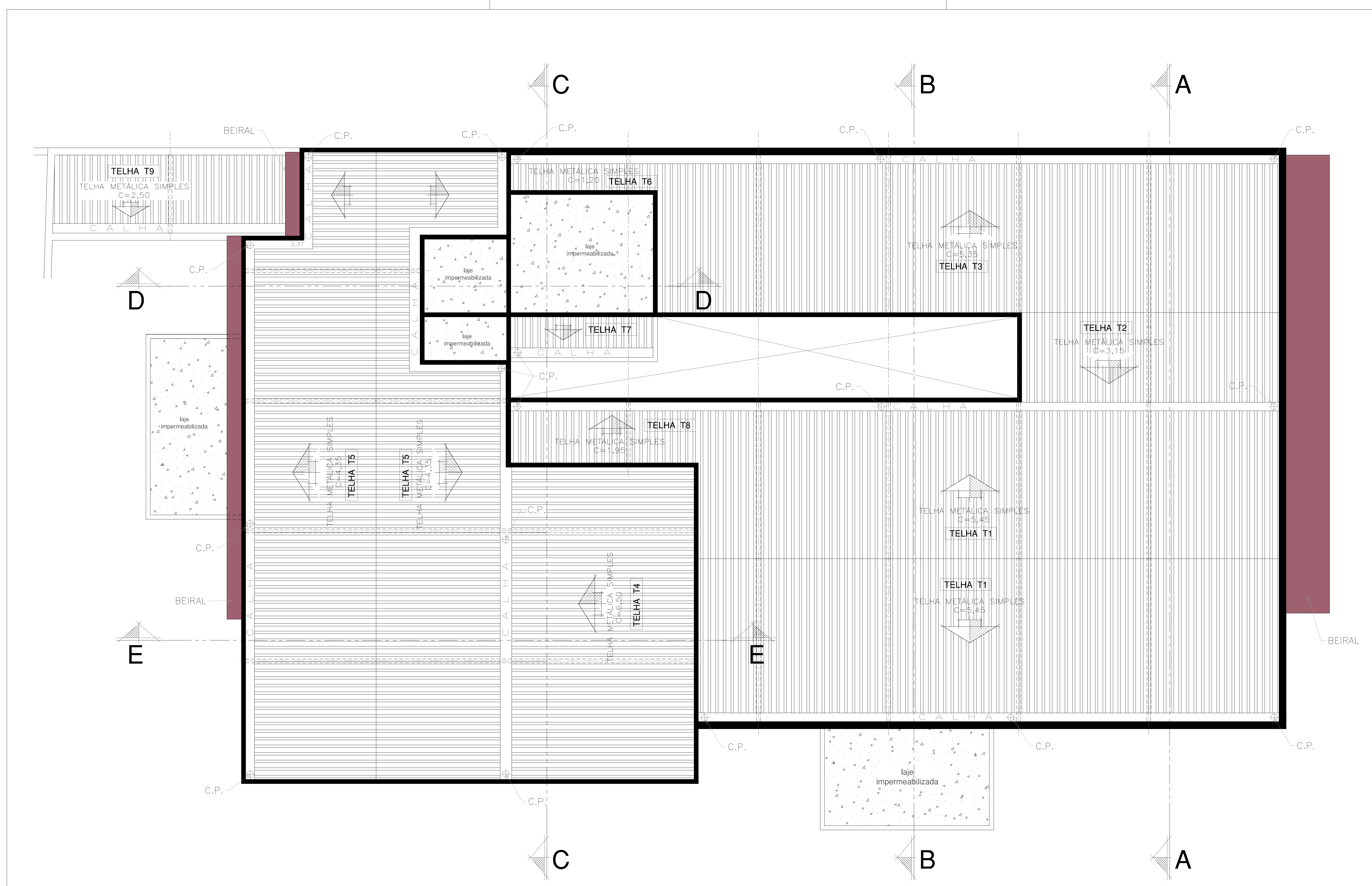
PLANTA DE LOCAÇÃO DAS TELHAS ESC.: 1:100
